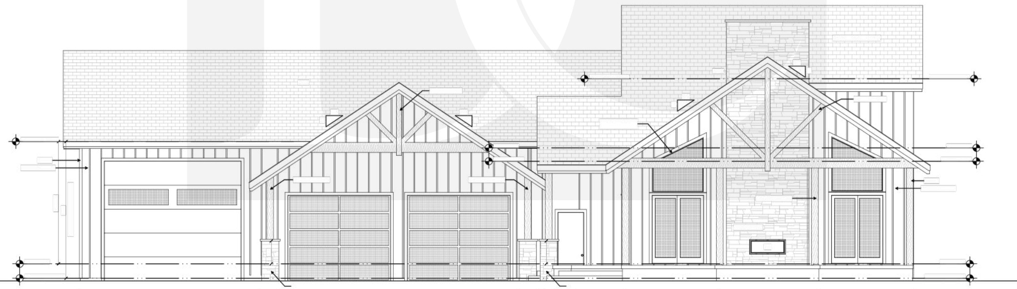
RIGHT ELEVATION
