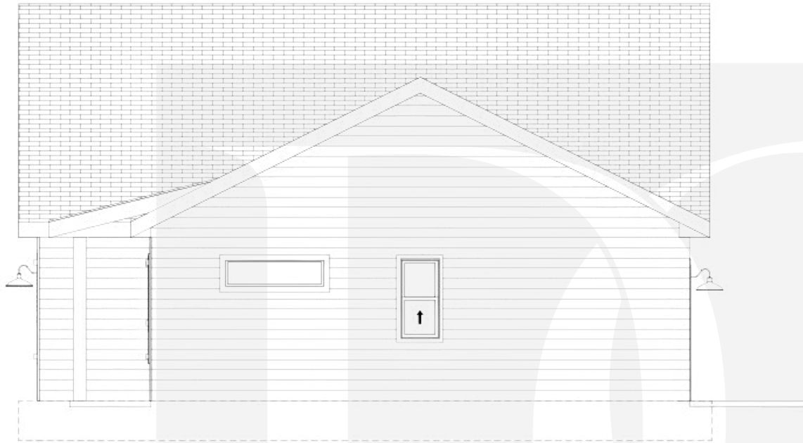
RIGHT ELEVATION
